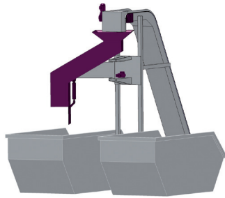
Containerbefüllung mittels Drehrutsche
