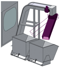
Dezentrale Schrottentorgung für Einzelpressen
