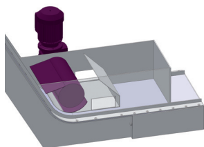
p.m. Rutschförderer mit Trichter und Separierwalze
