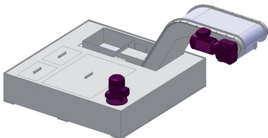
p.m. Rutschförderer Typ 125.4 mit Kühlmittelbehälter, Pumpe und Niveauregelung
