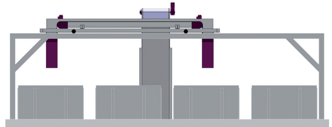
Containerbefüllung über fahrbaren Reversierförderer mit Schwenkrutschen
