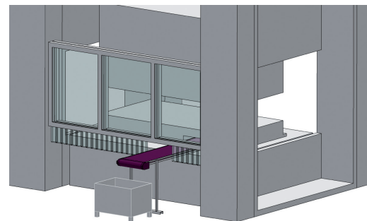
Beispiel: Schrottsorgung aus dem Werkzeug mit p.m. Gurtbandförderer
